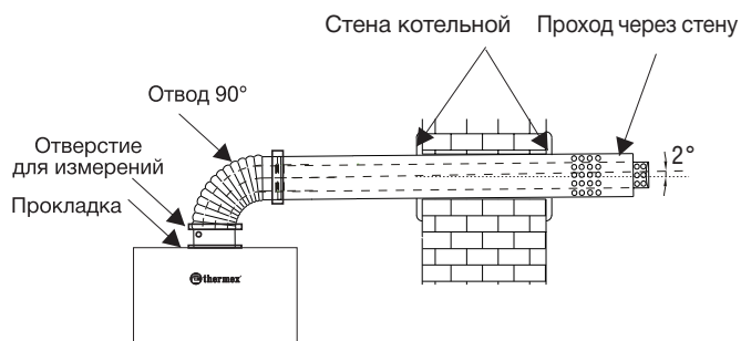
Рис. 5 Коаксиальный проход через стену
