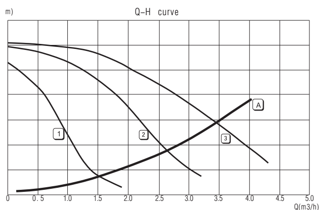
Рис.18 График производительности насоса и потери напора в котле (65кВт)
