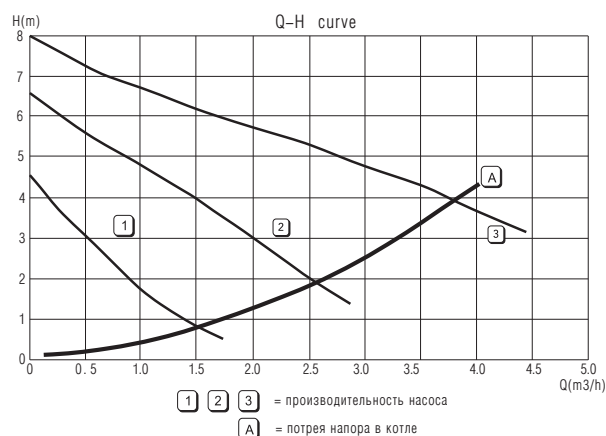
Рис.19 График производительности насоса и потери напора в котле (50кВт)
