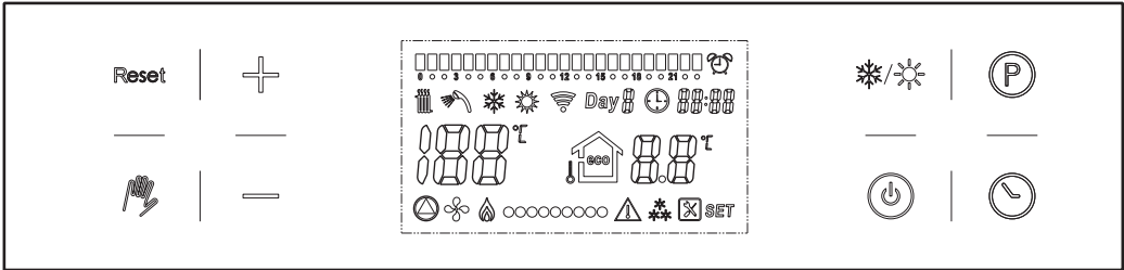
Рис. 12 Панель управления
