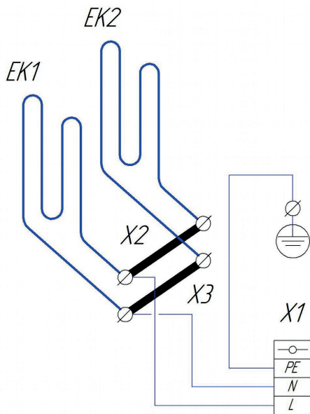
Рисунок 6 - Схема электромонтажная
