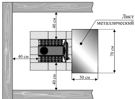
Рисунок-3. Установка отопительной печи.
