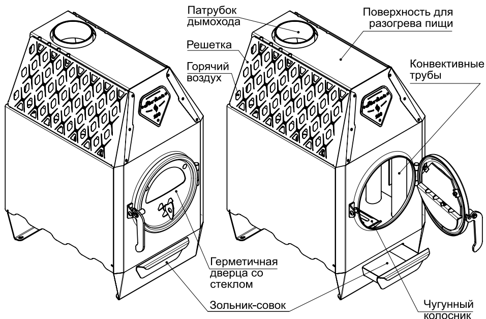
Рисунок - 1. Конструкция печи Stoker TERMO
