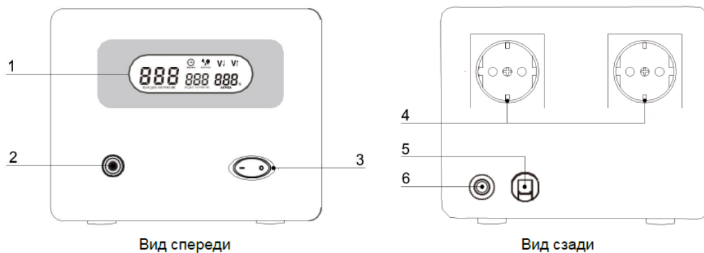
Рисунок 2. Внешний вид стабилизаторов напряжения SMARTWATT AVR TOWER 1500-2000VA. Описание элементов приводится в таблице 2.
