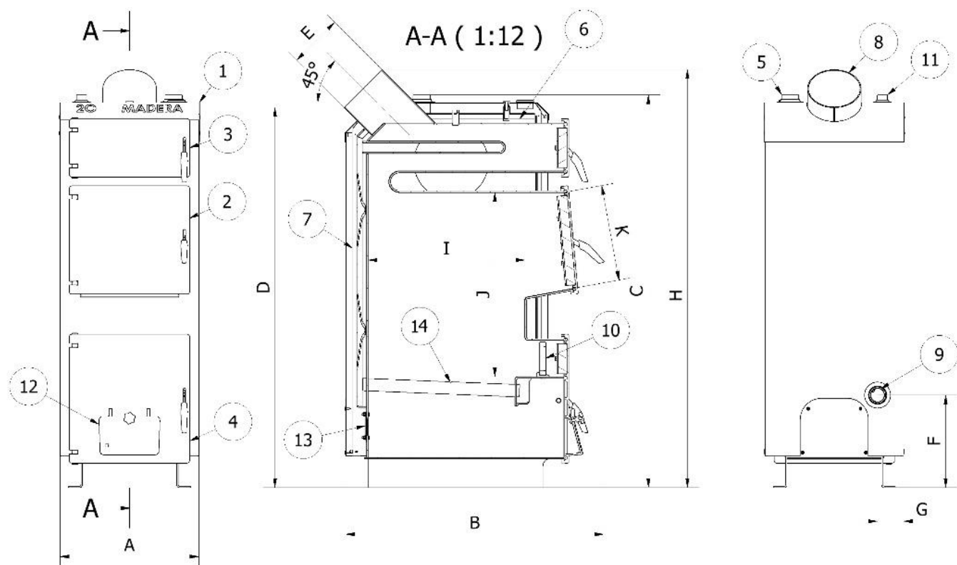
Рис 2. Схема котла SAKOVICH MADERA
