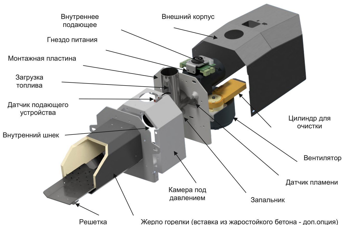
Рисунок 6. Состав Горелок Lавого Eco 16-102
