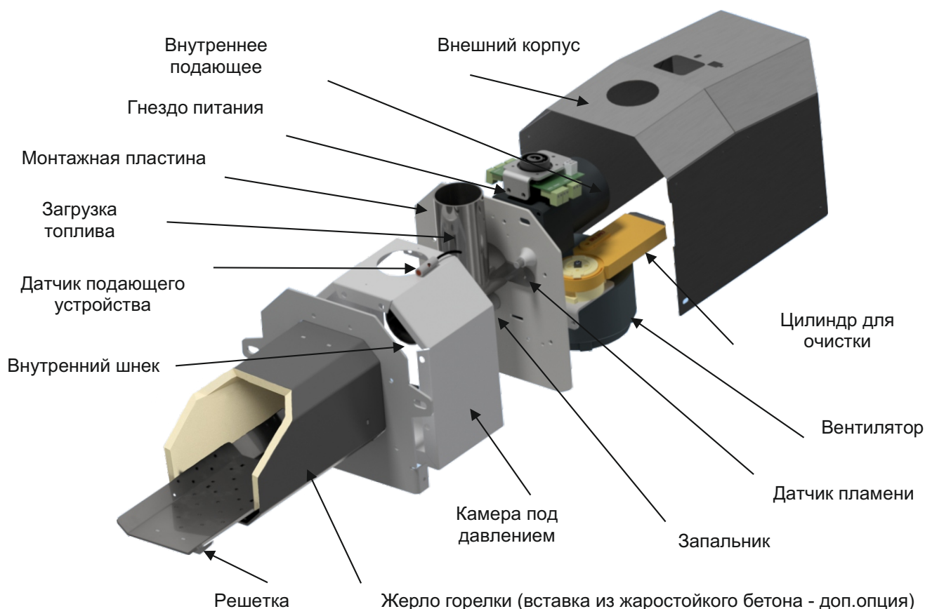
Рисунок 6. Состав Горелок Lavo Eco 16-102
