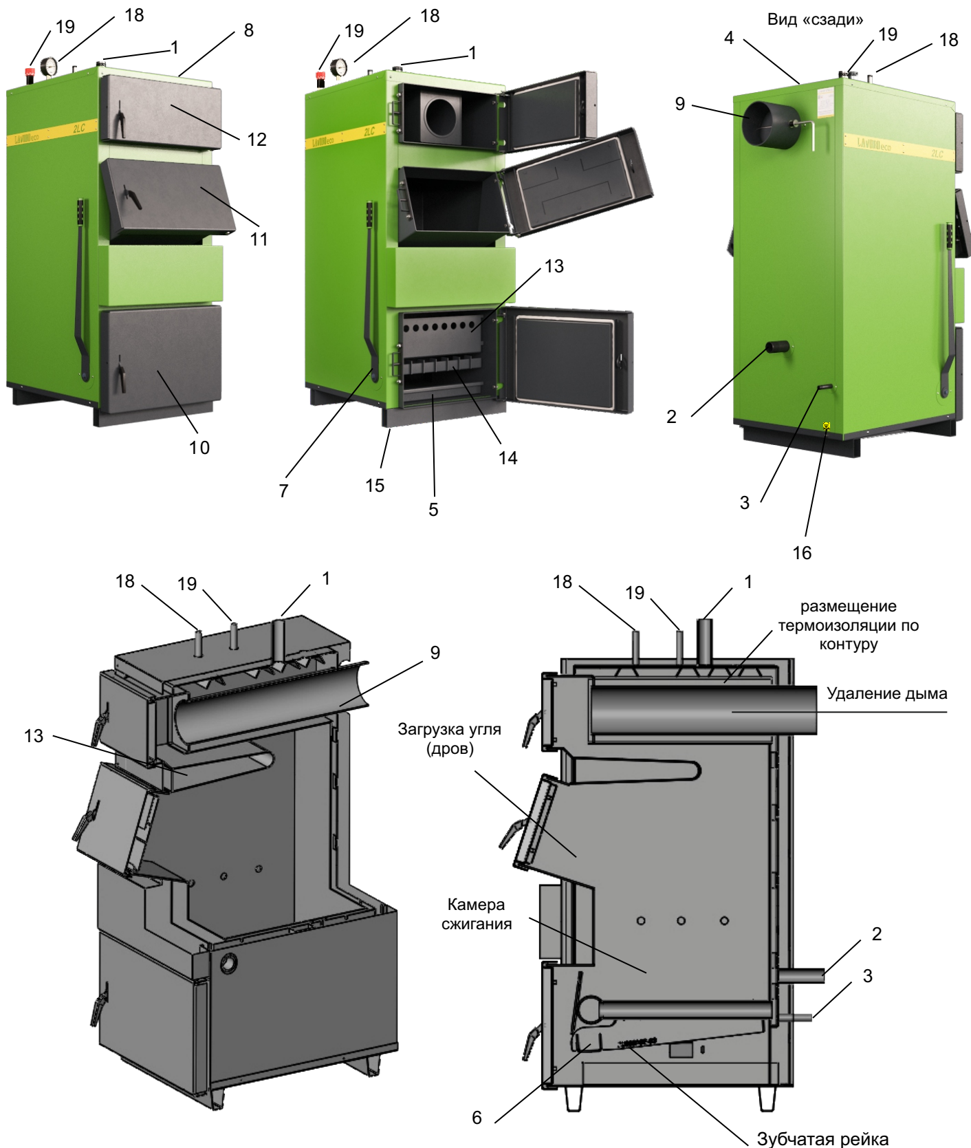
Рисунок 2. Состав и устройство Котлов моделей LC Mega 12-22 (в котле серии LC Mega 32 в верхней части топки добавлена еще одна водоуполненная полка)
