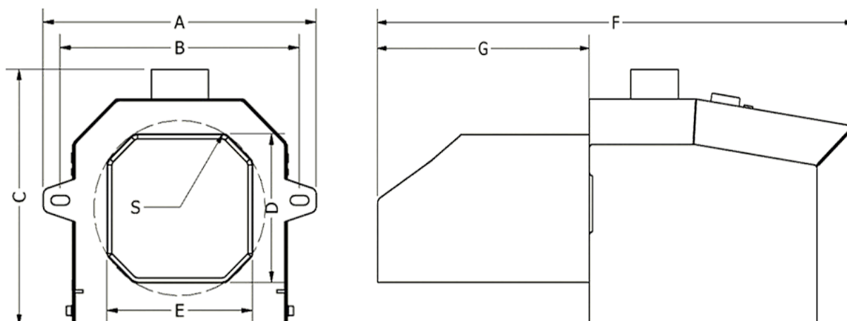
Рисунок 5. Габаритные и присоединительные размеры Горелок Lavoro Eco 16-99
