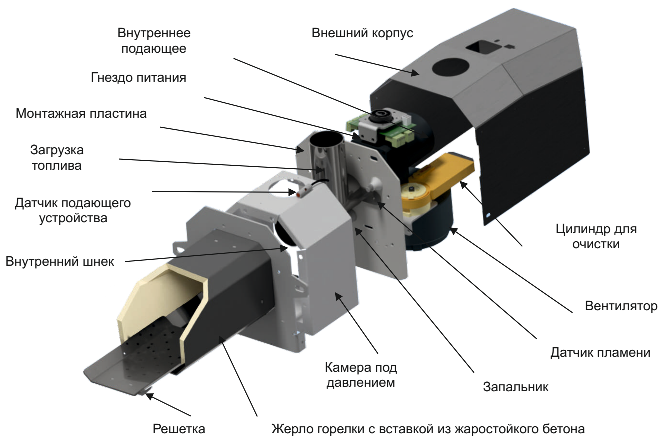
Рисунок 5. Состав Горелок Lavoro Eco 16-99
