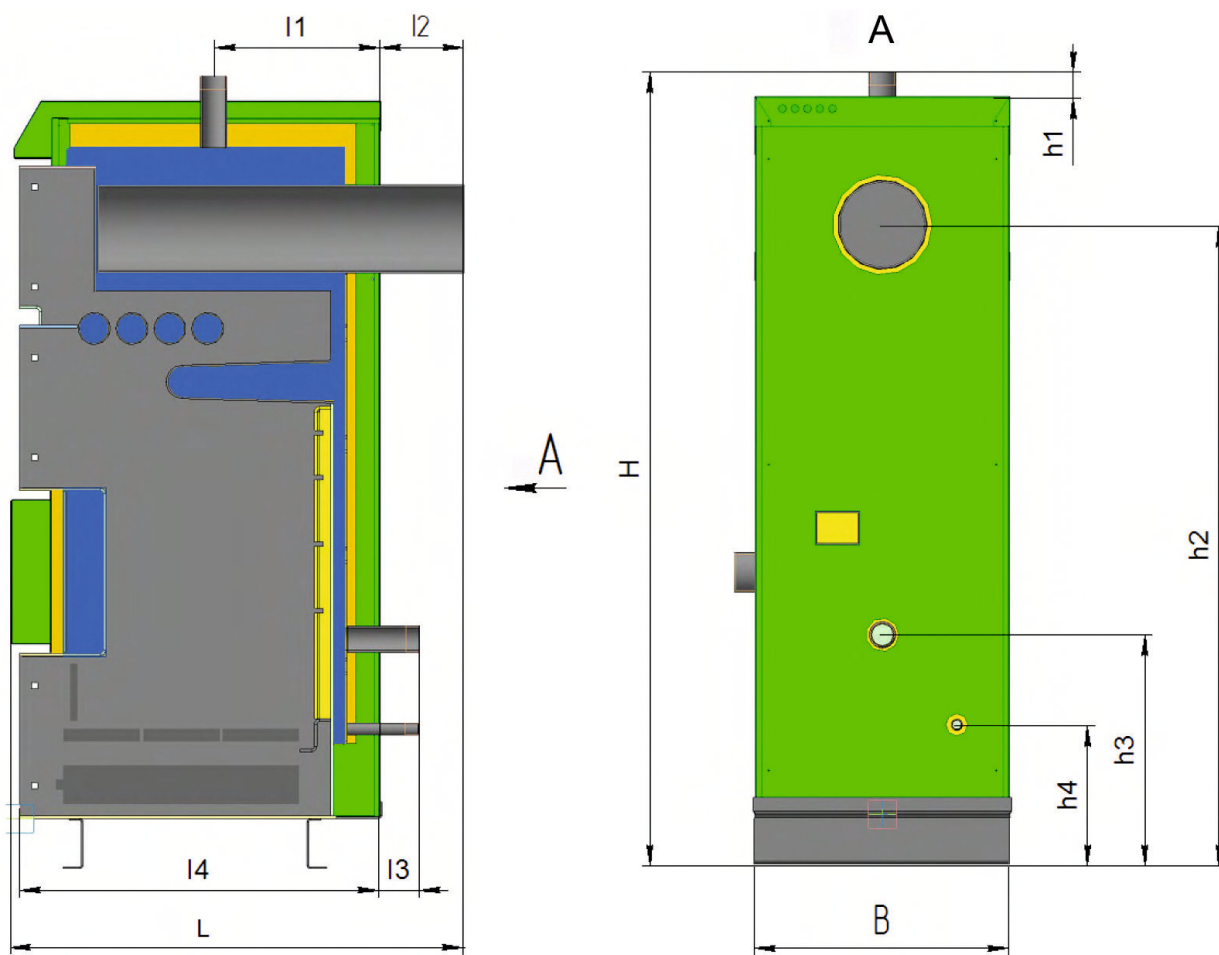
Рисунок 1. Габаритные и присоединительные размеры Котлов модели L-62, 82
