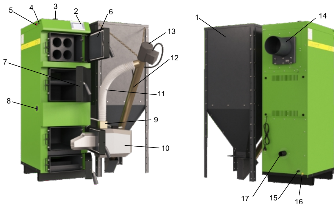
Рисунок 1. Состав и устройство Котлов моделей LF16-32
