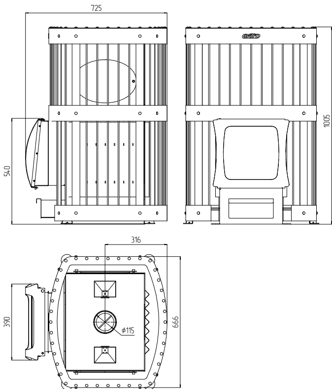
Рис. 2 Размерные характеристики печи «Grill'D» Fortuna 280 G short
