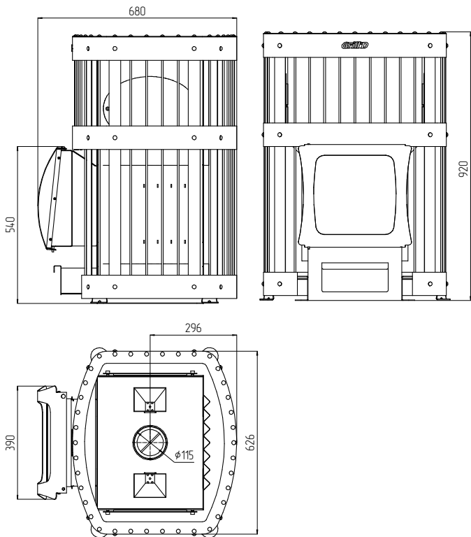
Рис. 1 Размерные характеристики печи «Grill'D» Fortuna 200 G short
