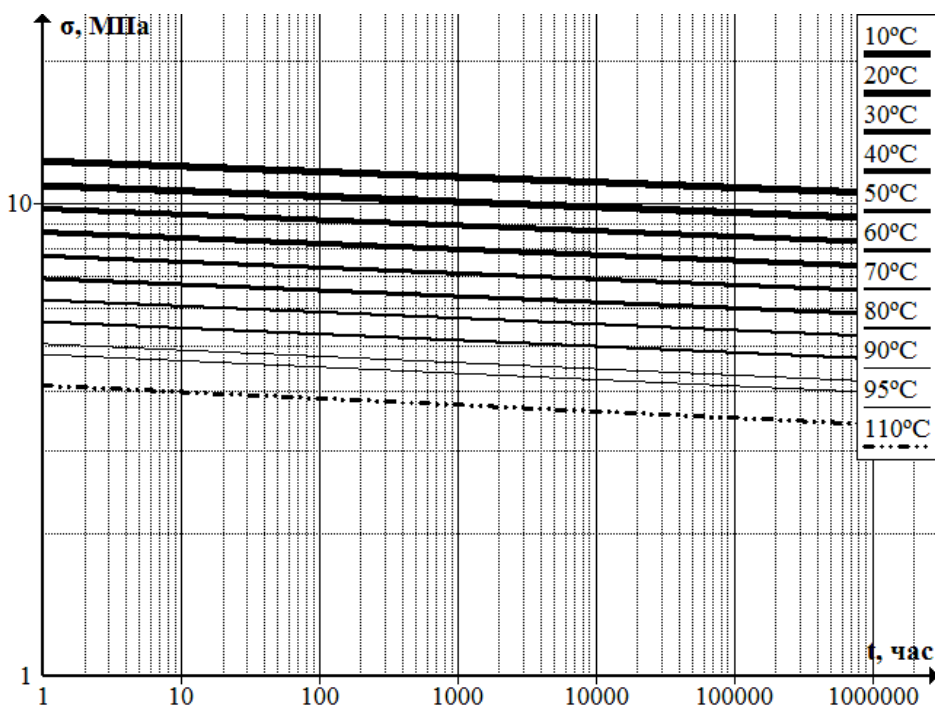
Рисунок 1 – Графики длительной прочности труб FED PE-Xa при различных температурах теплоносителя (σ – кольцевые напряжения; t – время работы до разрушения трубы)
