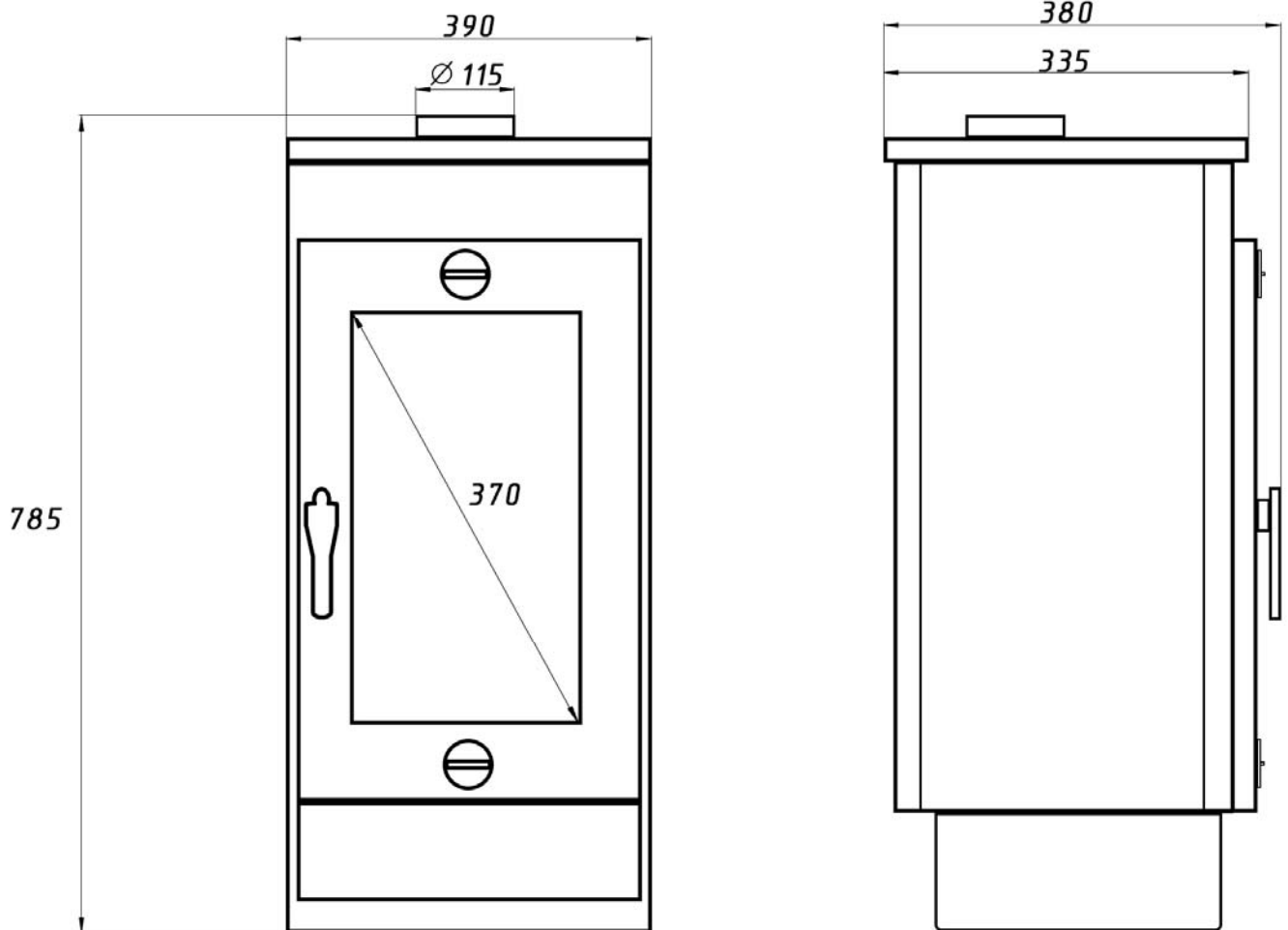
Схема печь-камин Ингода
