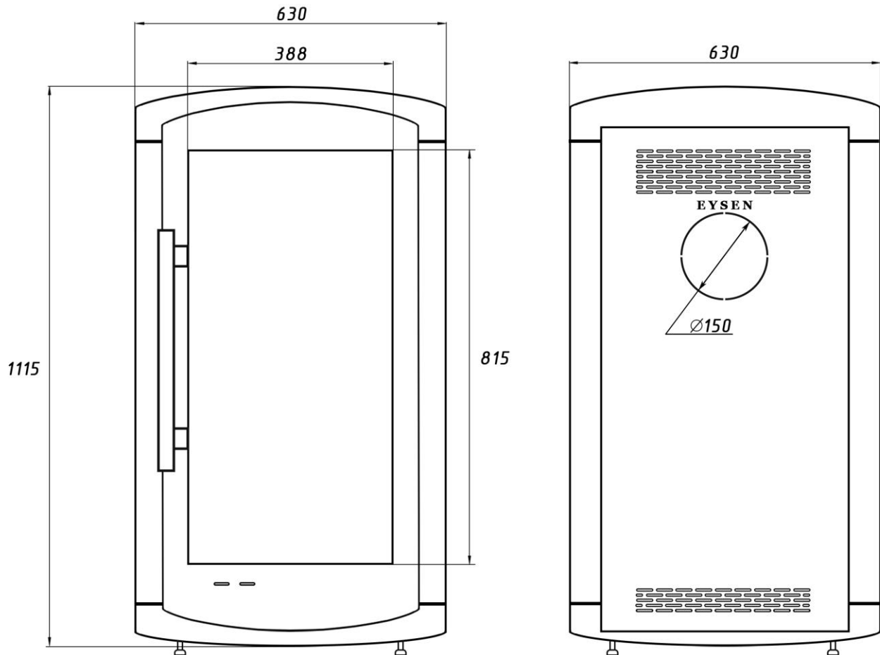
Схема печь-камин Royal Stone
