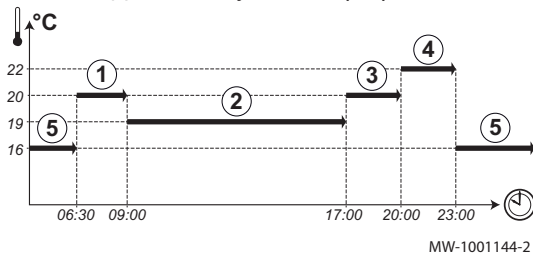
Рис.5 Действия суточной программы
