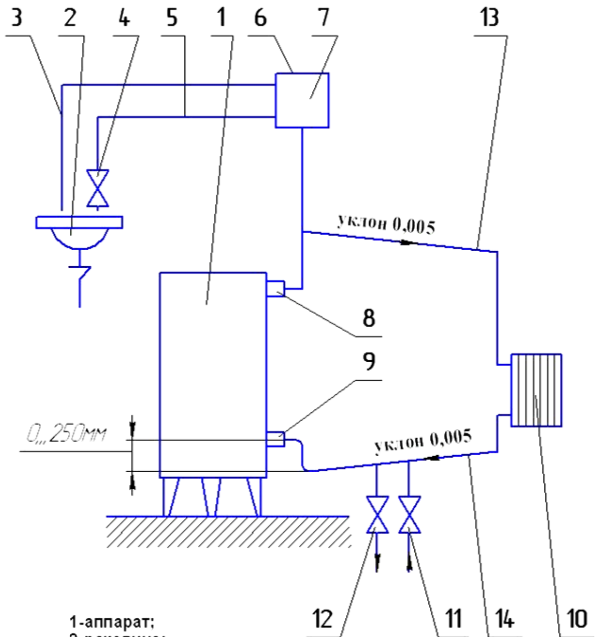
Рис.6 Схема присоединения аппарата к системе отопления.
