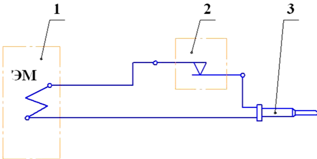
Рис.3 Схема электрическая.
