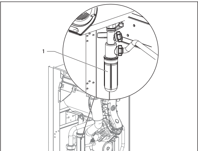
Рис. 5.2 Заполнение сифона
