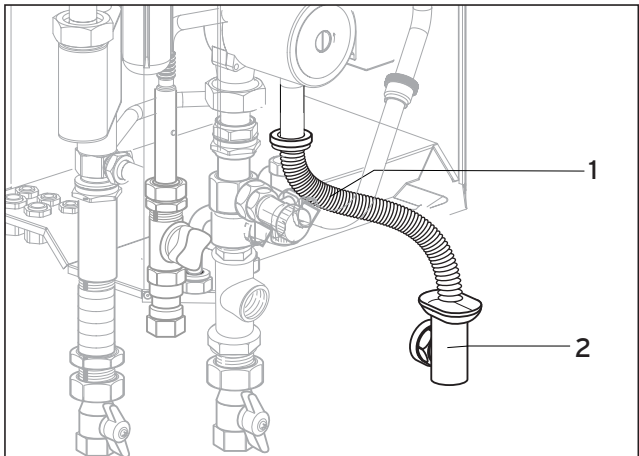
Рис. 4.9 Отвод конденсата
