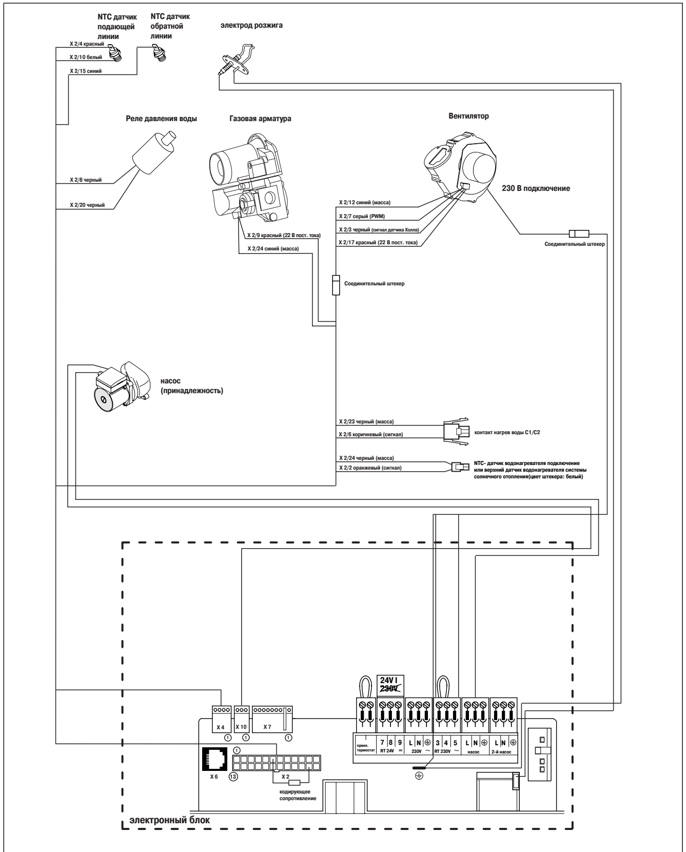
Рис. 4.12 Монтажная схема аппарата есоТЕС VU 466
