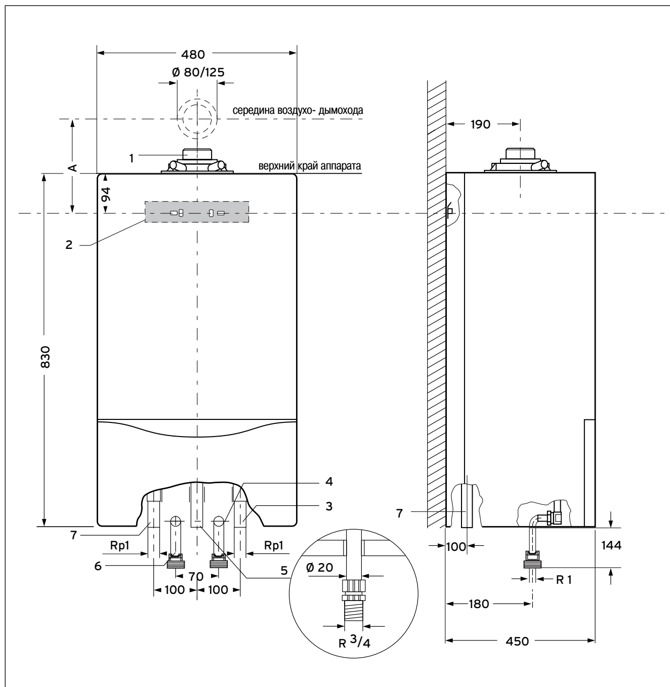
Рис. 3.2 Присоединительные размеры
