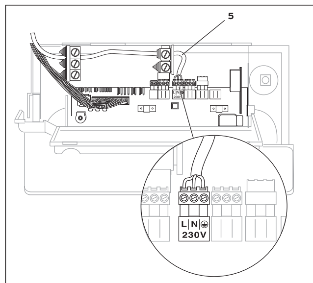
Рис. 4.10 Пример ввода кабеля
