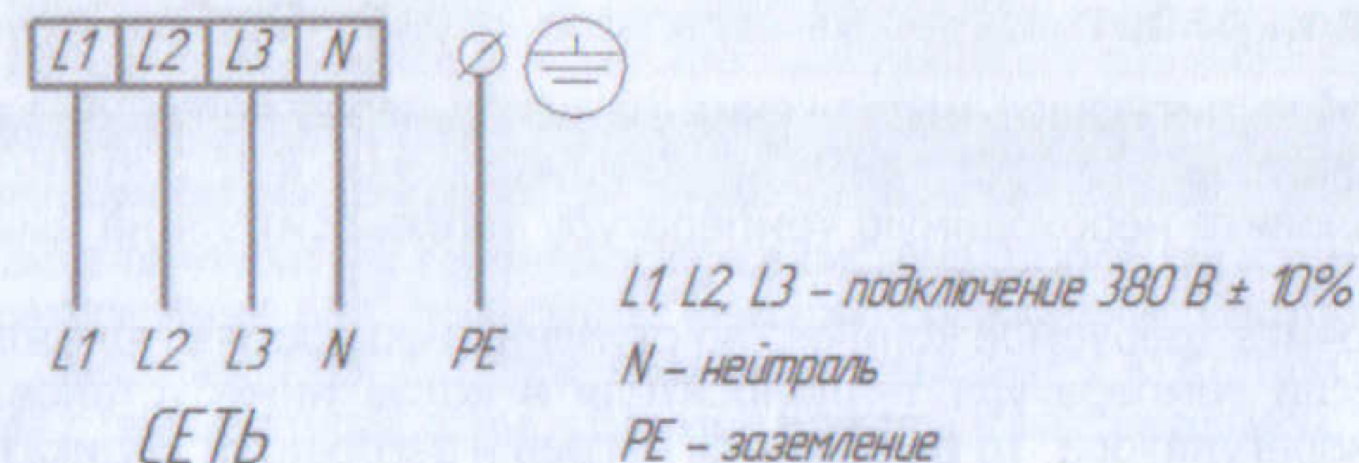
Рис. 4. Схемы подключения электрического котла к трехфазной электросети
