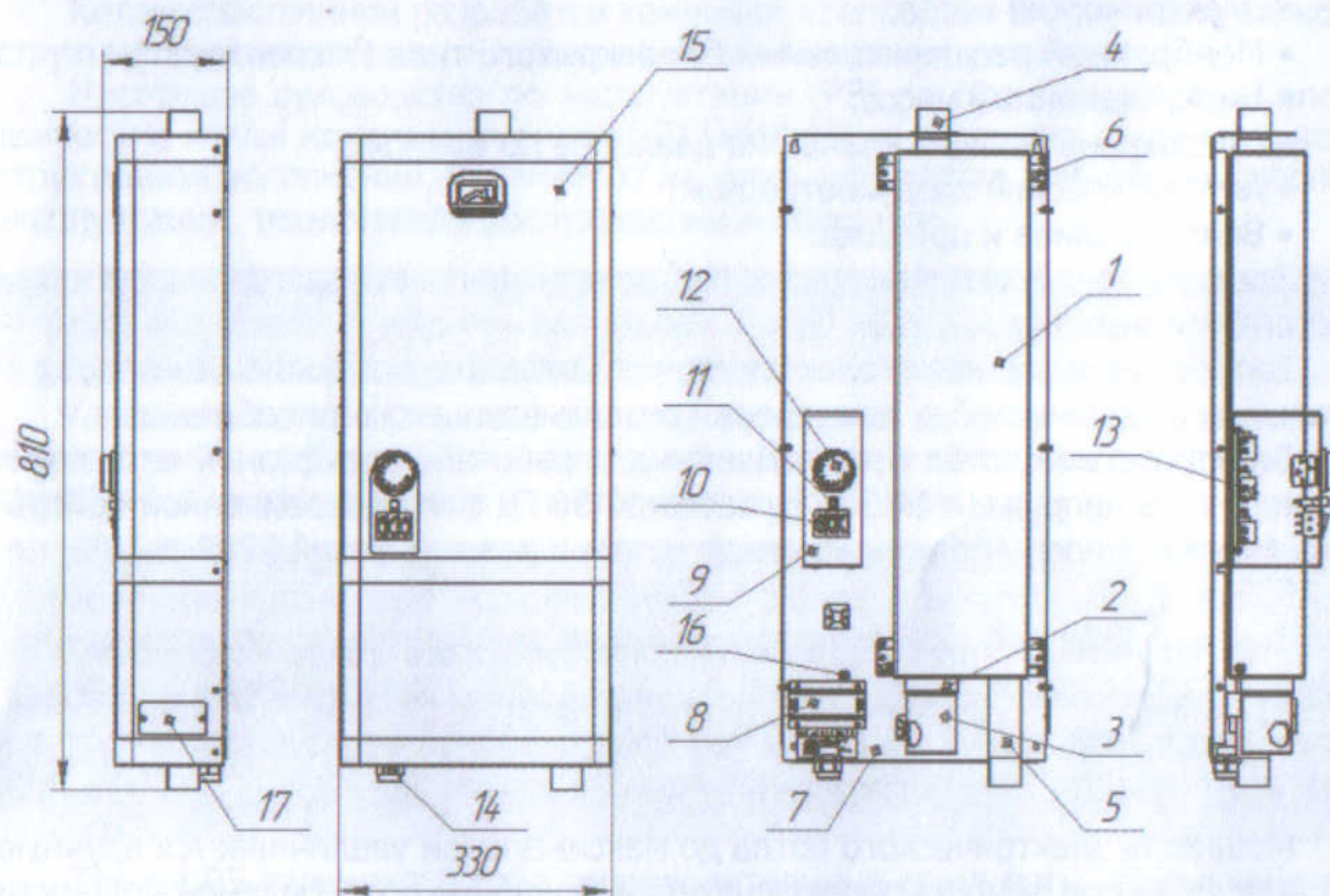
Рис. 1. Конструкция электрического котла «Спутник 15»
