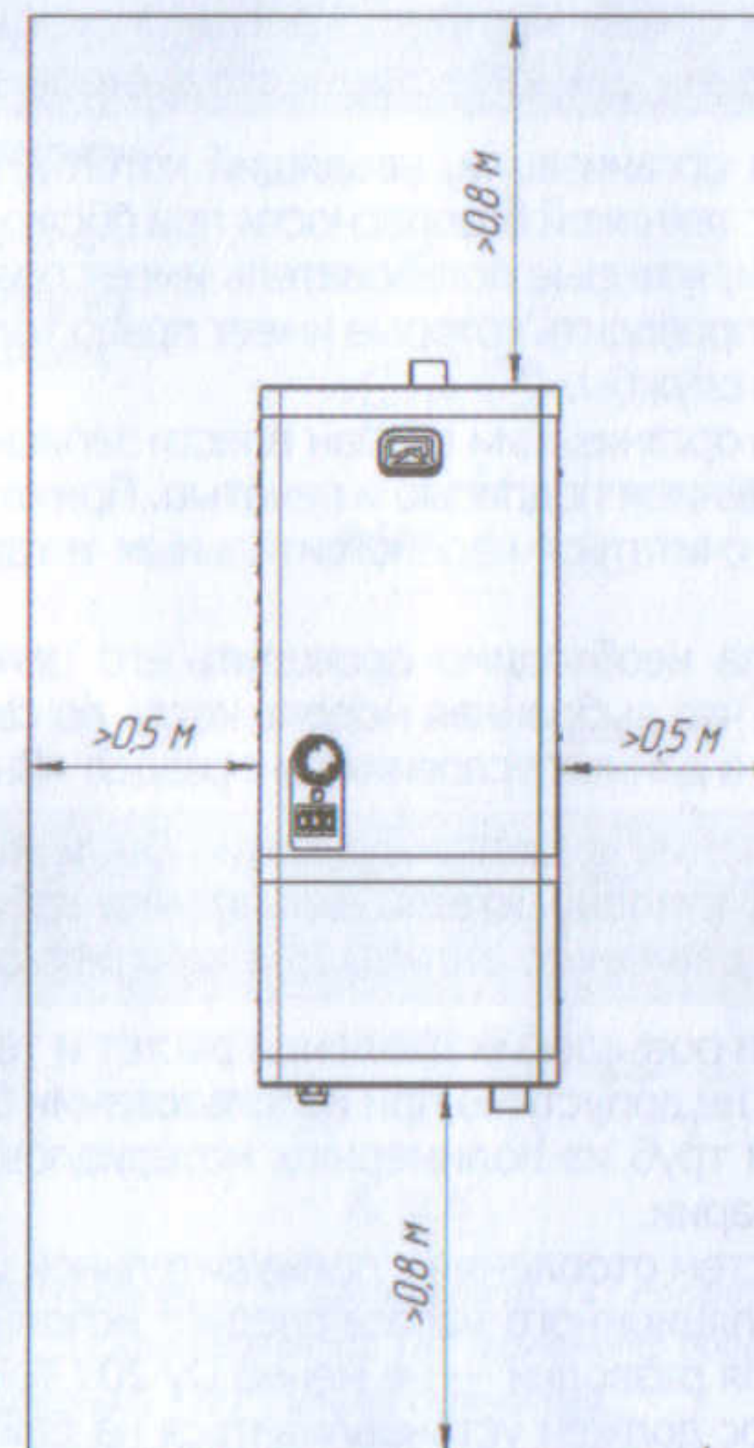
Рис. 2. Схема размещения котла в помещении.
