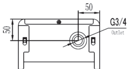
Рисунок 4.1. Габаритные размеры для подключения к системе отопления ECO-3, ECO-4,5.
