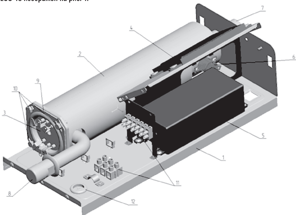
Рисунок 1. Котел отопительный электрический ECO-3, ECO-4,5, ECO-6, ECO-7,5, ECO-9, ECO-12, ECO-15, ECO-18
