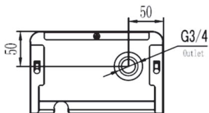
Рисунок 4.2. Габаритные размеры для подключения к системе отопления ECO-6, ECO-7,5, ECO-9, ECO-12, ECO-15, ECO-18.
