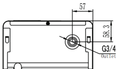
Рисунок 4.3. Габаритные размеры для подключения к системе отопления ECO-15, ECO-18.
