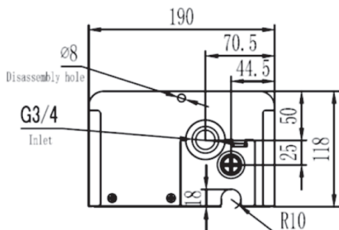
Рисунок 4.2. Габаритные размеры для подключения к системе отопления ECO-6, ECO-7,5, ECO-9, ECO-12, ECO-15, ECO-18.
