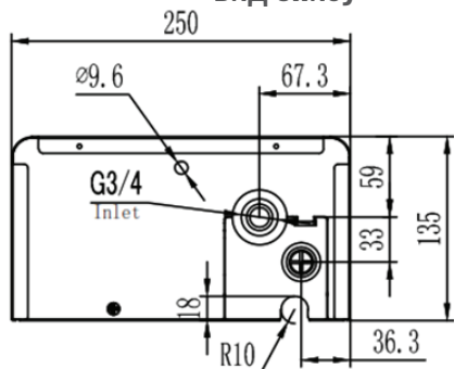
Рисунок 4.3. Габаритные размеры для подключения к системе отопления ECO-15, ECO-18.
