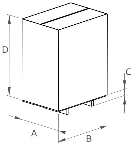
Схема 3. Габаритные размеры котла и поддона, модель WBS Ligna 50
