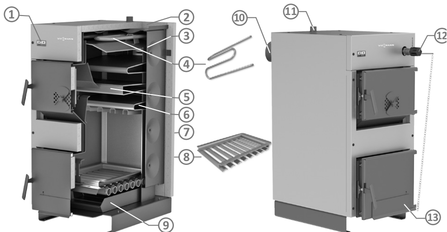
Схема 11. Элементы котла WBS Ligna 50
