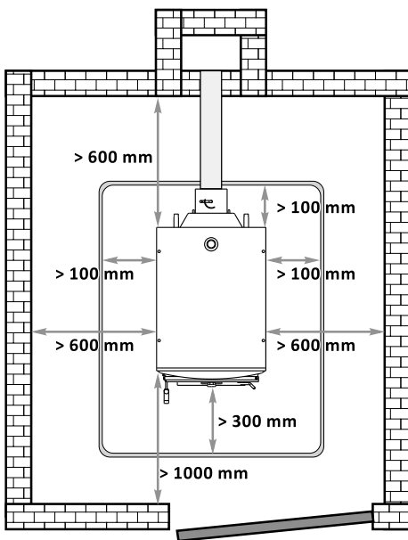
Схема 1. Рекомендуемое расстояние от котла до стен
