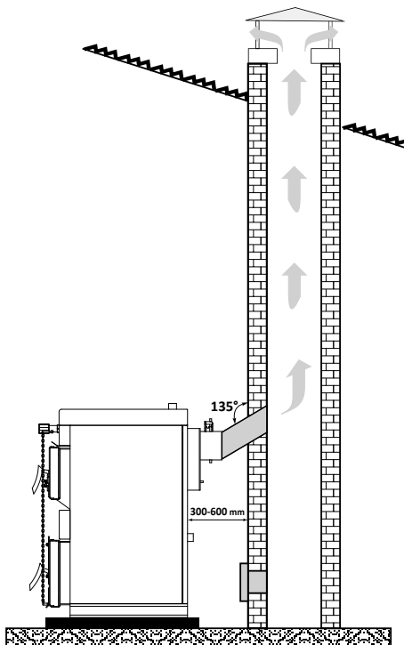
Схема 4. Зависимость между мощностью котла и параметрами дымохода
