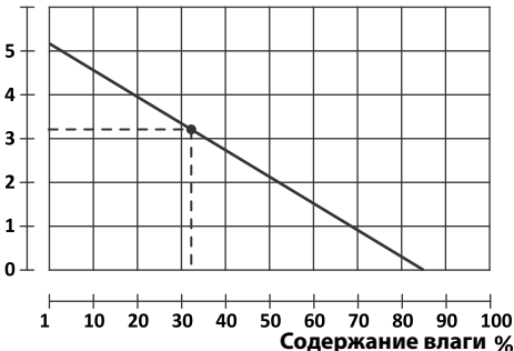
Схема 2. Зависимость калорийности древесины по отношению к влаге в ней
